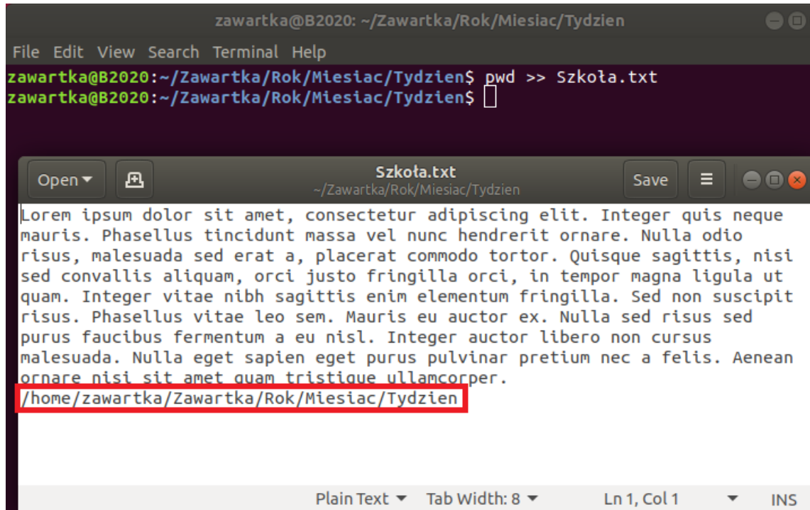
Obrazek 5: Wrzucenie ścieżki katalogu Tydzien na koniec pliku Szkoła.txt
