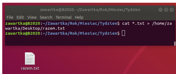
Obrazek 15: Działanie polecenia cat *.txt
