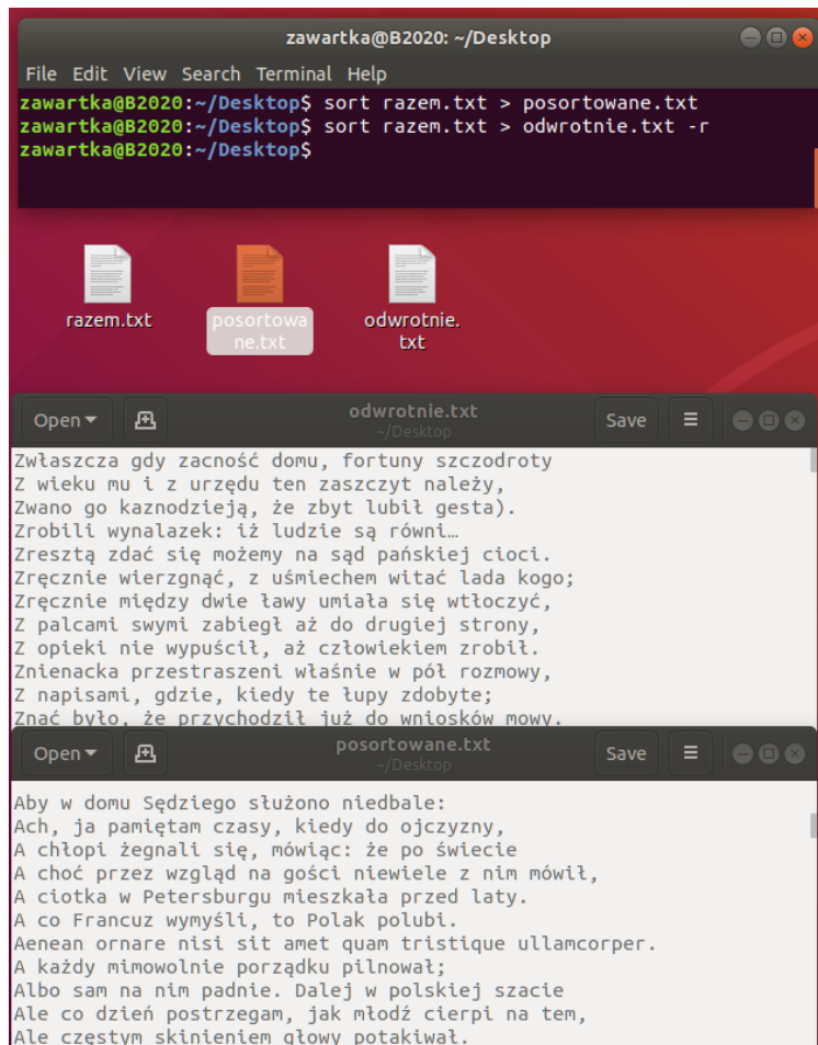
Obrazek 16: Efekt polecenia sort
