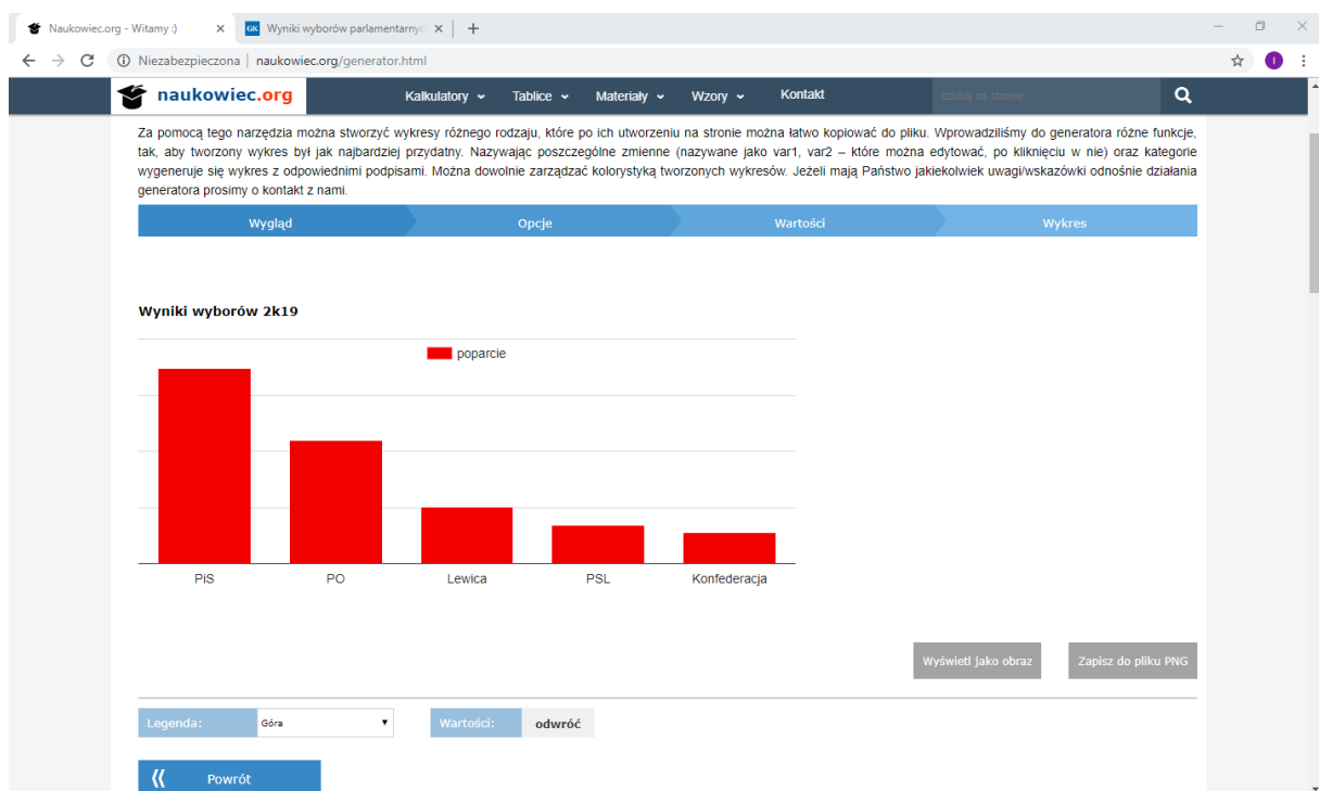
Obrazek 4: Przykładowy wykres wygenerowany przy użyciu strony naukowiec.org
